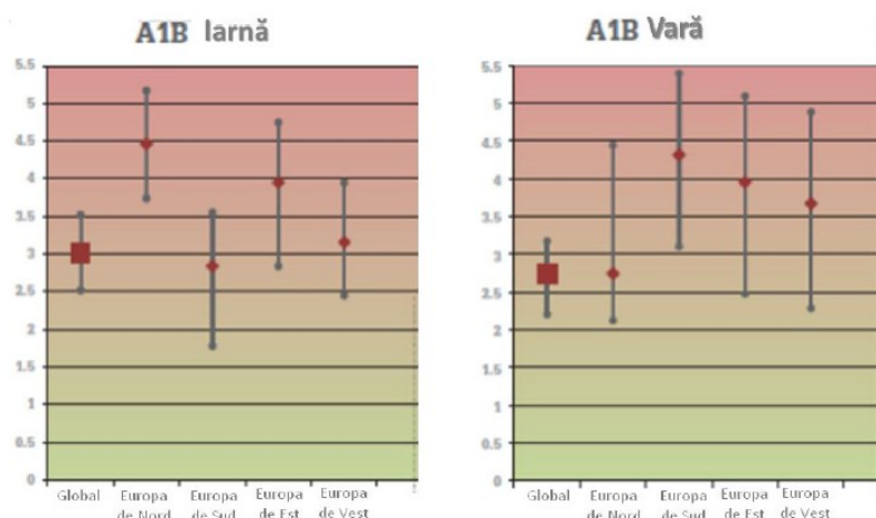
Figura 19: Modificări ale temperaturii în diverse regiuni ale Europei
