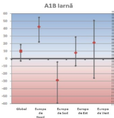
Figura 20: Modificări ale precipitațiilor în diverse regiuni ale Europei
