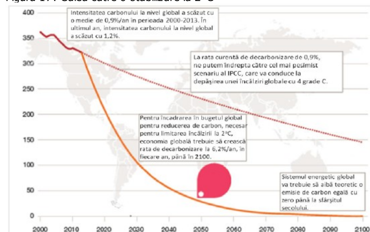
Figura 17: Calea către o stabilizare la 2°C
