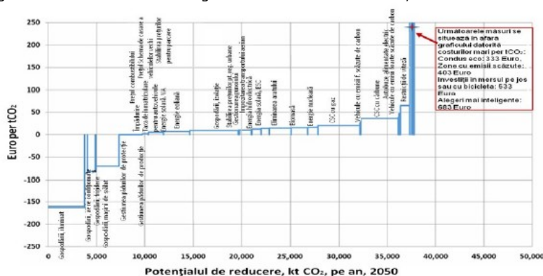
Figura 1: Curba costurilor marginale de reducere a emisiilor, la nivel transectorial, 2050
