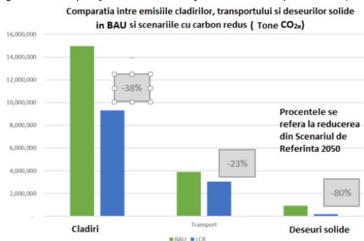
Figura 11: Comparație a Emisiilor BA U și a Scenariilor LC pentru clădiri, transport și deșeuri solide
